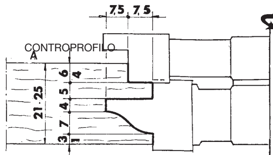
ESEMPI DI PROFILI - EXAMPLES OF PROFILES - BEISPIELE VON PROFILEN
