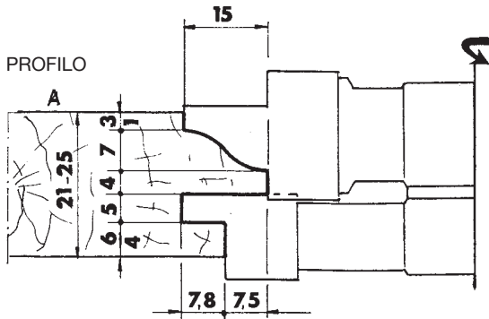
ESEMPI DI PROFILI - EXAMPLES OF PROFILES - BEISPIELE VON PROFILEN
